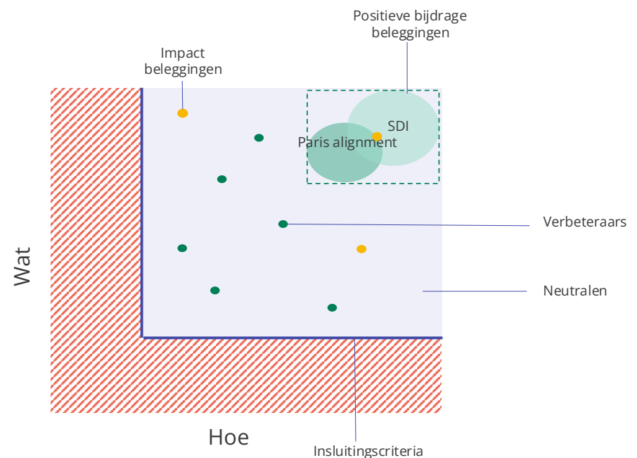
Figuur 2: Duurzaamheidsraamwerk
